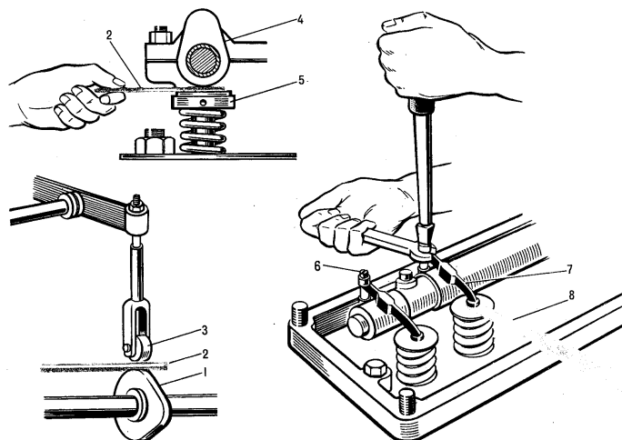
Рисунок 7 - Проверка и регулировка теплового зазора в клапанном приводе где, 1-кулачная шайба, 2-измерительный щуп, 3-ролик толкателя, 4 - кулачная шайба, 5- тарелка упорная, 6-регулирующий винт, 7-клапанный рычаг, 8-щуп.
