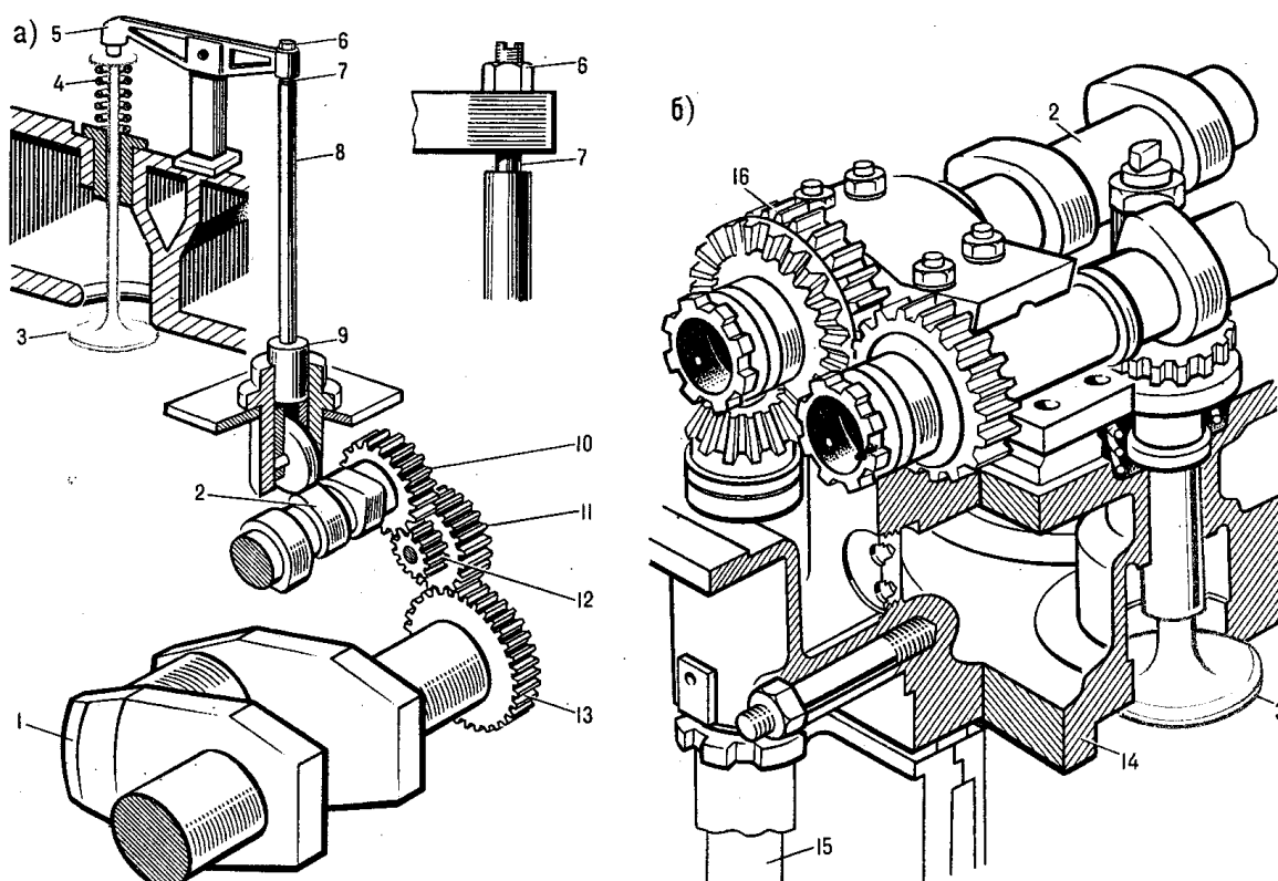
Рисунок - 4 Клапанные приводы с нижним и верхним расположением распределительного вала
