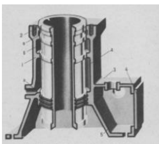
Рис. 11. Блок цилиндров двигателя Г74
