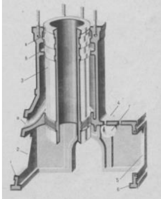
Рис. 11. Блок цилиндров двигателя Г74
